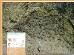
枕状溶岩
